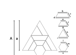
A 34,1 cm - 13 3/8" B 33,7 cm - 13 1/4" a 29,2 cm - 11 1/2" b 11,2 cm - 4 3/8" c 5,4 cm - 2 1/8" d 16,7 cm - 5 5/8" e 5,5 cm - 2 1/8" f 5,4 cm - 2 1/8" g 11 cm - 4 3/8" h 11 cm - 4 3/8" i 11 cm - 4 3/8" l 11 cm - 4 3/8" m 5,5 cm - 2 1/8" n 11 cm - 4 3/8"
