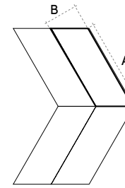
Chevron A 26,4 cm - 10 3/8" B 9,6 cm - 3 3/4"
