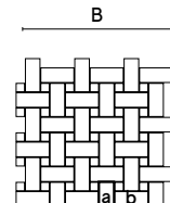
Basket Weave A 30,5 cm - 12" B 30,5 cm - 12" a 6,7x2,9 cm - 2 5/8"x1 1/8" b 1,7x1,7 cm - 5/8"x5/8"
