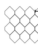
Mosaico Esagono 3D A 8,8 cm - 3 1/2" B 8,1 cm - 3 1/8"
